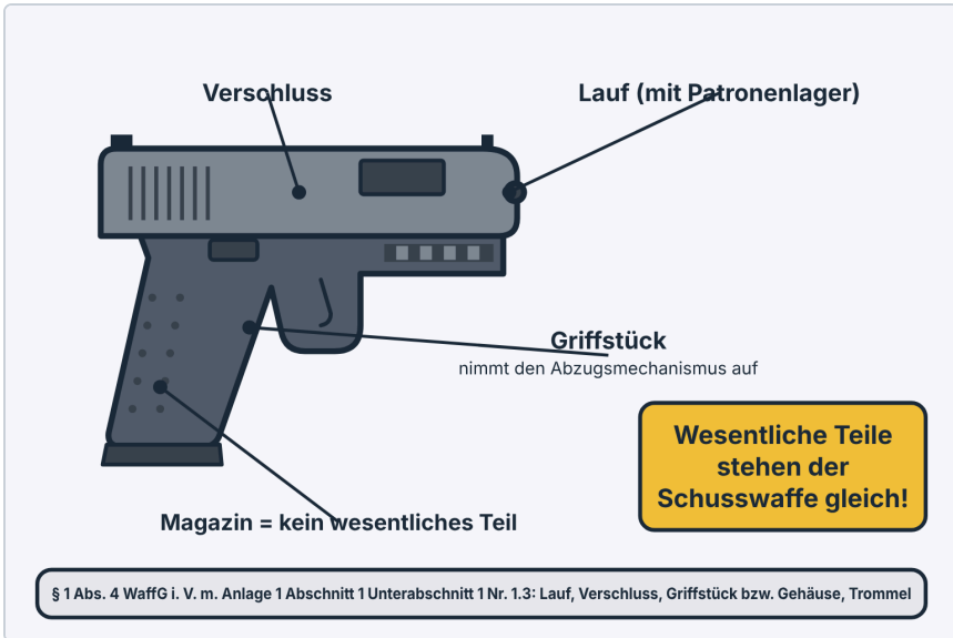
Abb. 4.1 Wesentliche Teile einer Selbstladepistole: Lauf (mit Patronenlager), Verschluss und Griffstück. Magazin, Schließfeder und Visierung sind keine wesentlichen Teile.
