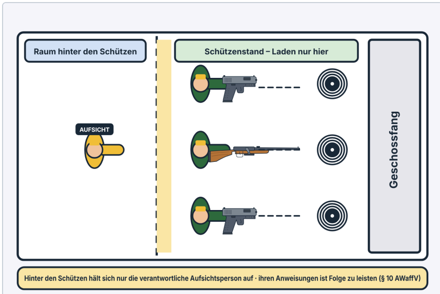
Abb. 26.3 Schießstand schematisch: Laden nur am Schützenstand, hinter den Schützen nur die Aufsicht.
