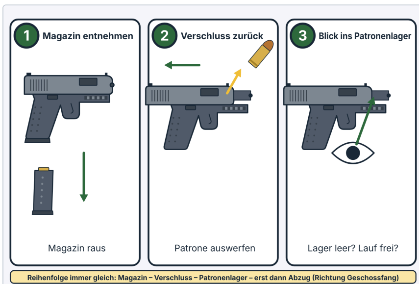
Abb. 26.2 Entladen und Prüfen einer Selbstladepestole: erst das Magazin, dann der Verschluss, dann der Blick ins Lager.
